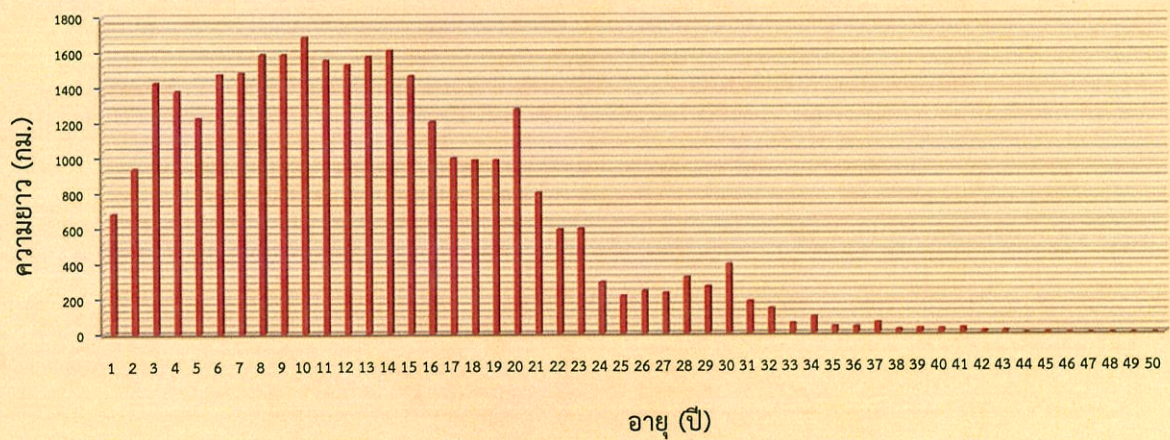
กราฟแสดงความยาวท่อจ่ายน้ำ Distribution Pipe (กม.) แยกตามอายุ
