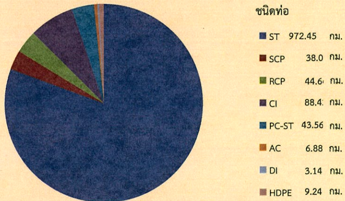
กราฟแสดงความยาวท่อจ่ายน้ำ Distribution Pipe (กม.) แยกตามชนิดท่อ
