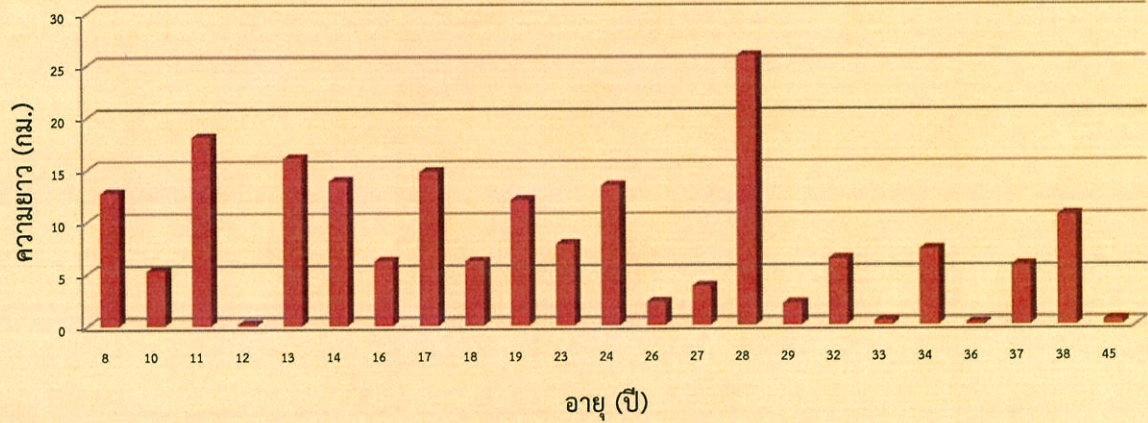
กราฟแสดงความยาวอุโมงค์ส่งน้ำ Tunnel and Conduit (กม.) แยกตามอายุ
