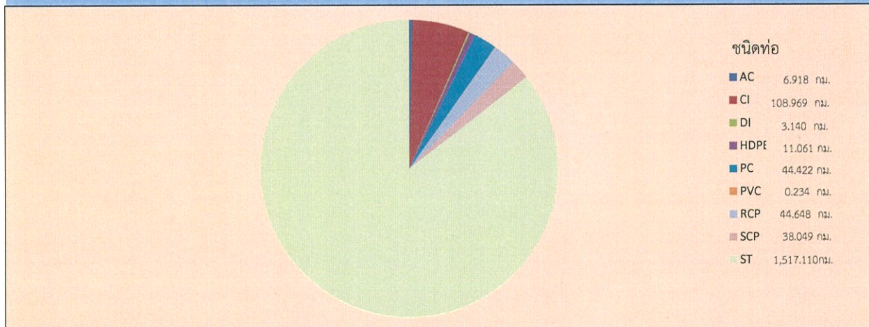
กราฟแสดงความยาวท่อประธาน Trunk Main (กม.) แยกตามชนิดท่อ
