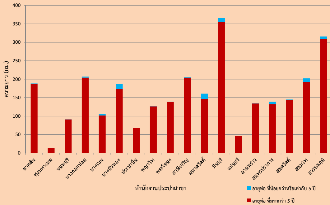
กราฟแสดงความยาวท่อจ่ายน้ำ (กม.) ชนิดซีเมนตีโยหิน ; AC แยกตามสำนักงานประปาสาขา
