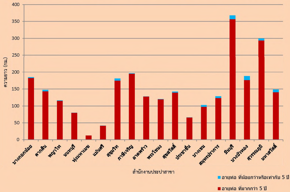
กราฟแสดงความยาวท่อจ่ายน้ำ (กม.) ชนิดซีเมนติโยหิน ; AC แยกตามสำนักงานประปาสาขา
