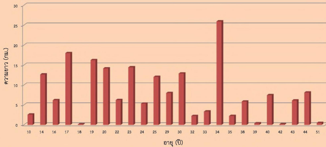
กราฟแสดงความยาวท่อประธาน Trunk Main (กม.) แยกตามอายุ
